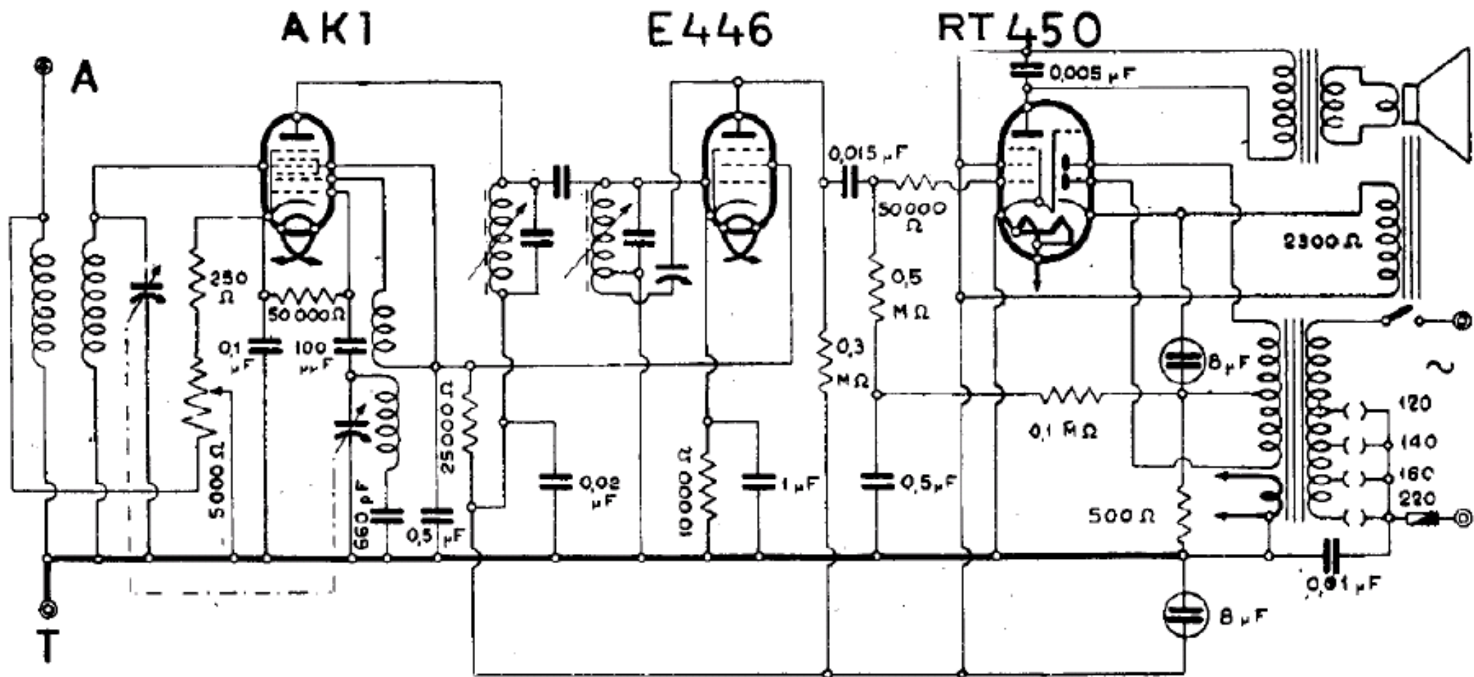
F.I.M.I. - MOD. PHONOLA « 670 M »
